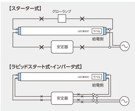
■ 工事結線図
