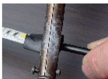
⑦熱伸縮チューブ取付
